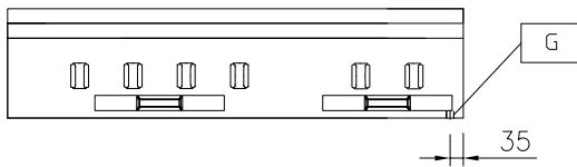
Front aanzicht
