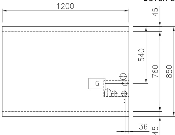
Boven aanzicht
